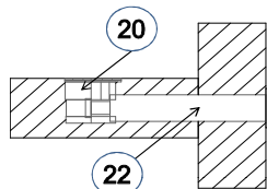
Эксцентриковая стяжка
