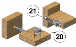
Эксцентриковая стяжка
