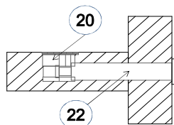
Эксцентриковая стяжка
